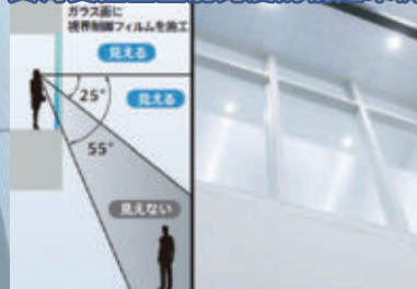
具有受控垂直能見度的構造示例
